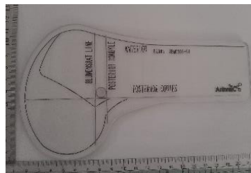
MPFLガイド (内側膝蓋大腿靱帯再建具)
