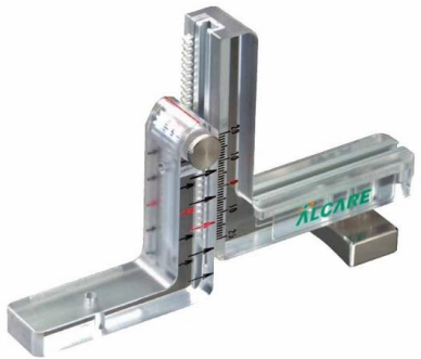
KMI (膝靱帯計測器)
